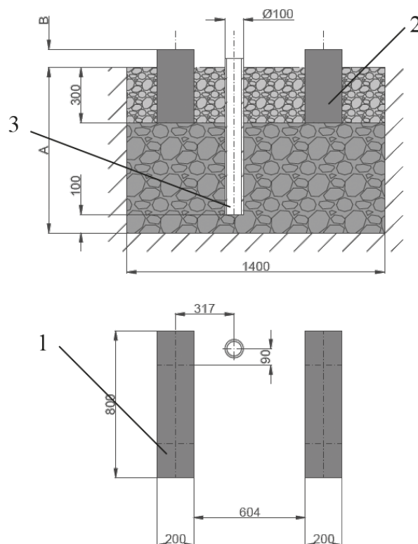
Tekening 7. Fundering voor de warmtepomp - bovenaanzicht
