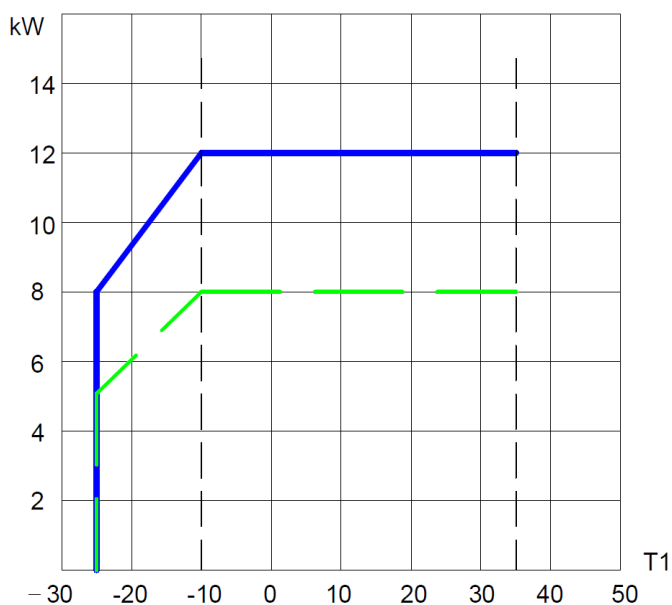
Tekening 4. Vermogensbereik warmtepomp Hti20/12 en HTi20/8
