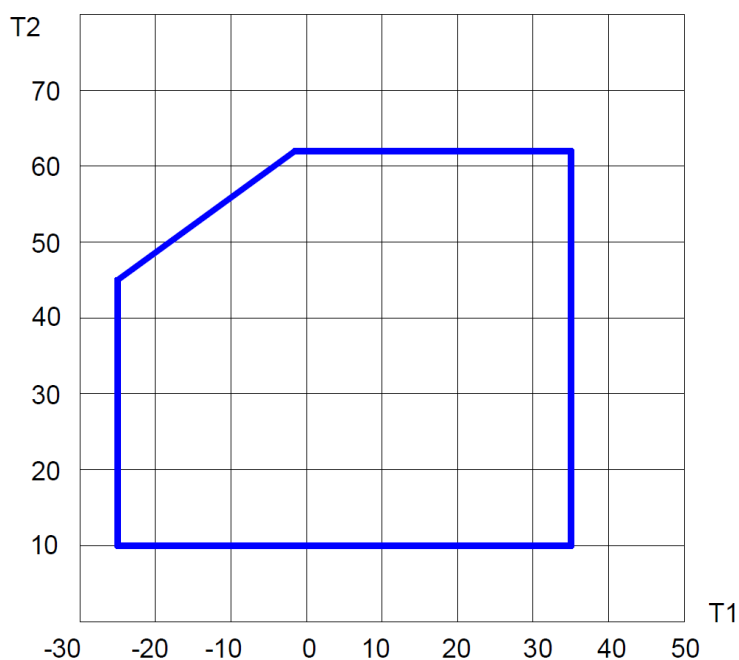
Tekening 3. Temperatuurbereik werklucht compressor
