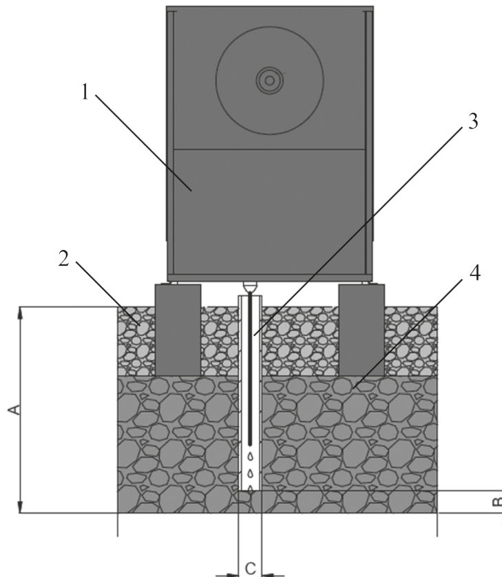
Tekening 6. Plaatsing en montage van de pomp
