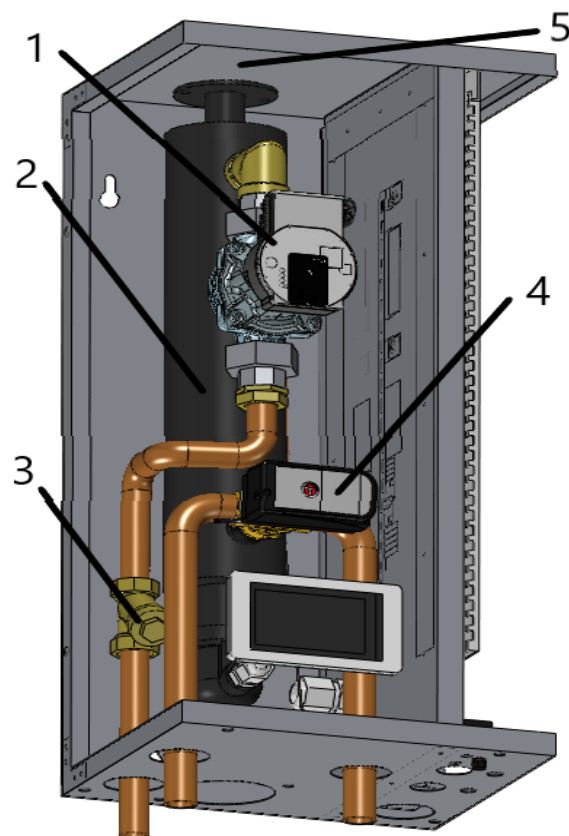
Tekening 10. Smart Binnenmodule
