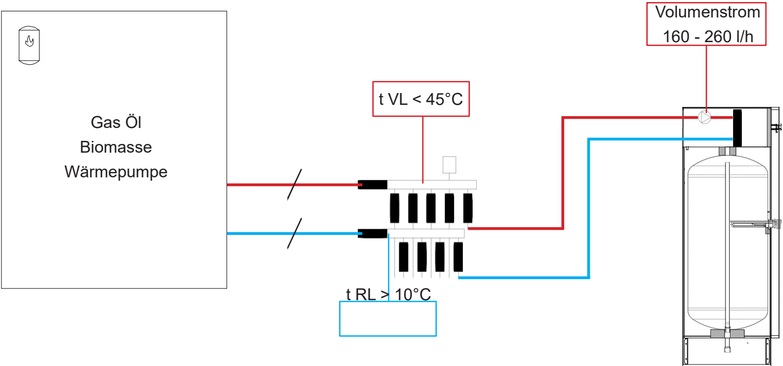
Schema 2 Anschluss an den Rücklauf Hauptstrang MFH oder nach FBH Verteiler
